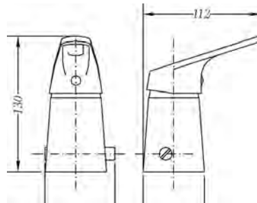
Ref.: 61142 22 45 66 Monomando de bidé con transmisión Single lever bidet mixer with diverter
