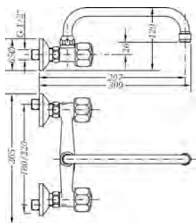
Ref.: 68104 11 45 66 Grupo mural fregadera 20 cm caño tubo alto 24cm Wall sink mixer 20cm high tube spout 24cm
