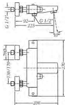
Ref.: 67100 26 45 67 Termostática de baño sin kit Thermostatic bath without kit
