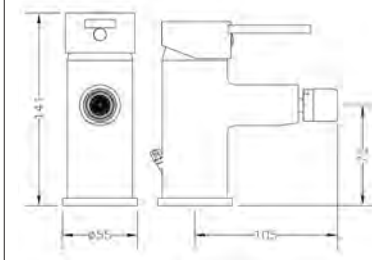
Ref.: 65145 29 45 66 Monomando de bidé Single lever bidet mixer
