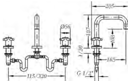
Ref.: 68120 08 45 66 Batería de lavabo caño recto Widespread wash basin mixer with straight pipe
