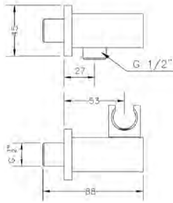
Ref.: 1649 04 Soporte ducha con toma cuadrado Square shower holder with flexible connector
