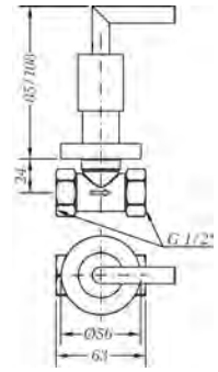
Ref.: 68170 12 45 66 Llave de paso 1/2" Stopcock 1/2"
