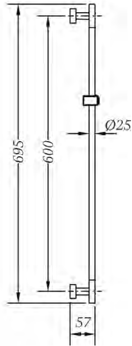
Ref.: 1747 45 Conjunto Kenjo, barra, flexo y ducha 3 jets (caja) Kenjo set, bar, flexible hose and 3 jets handshower (box)
