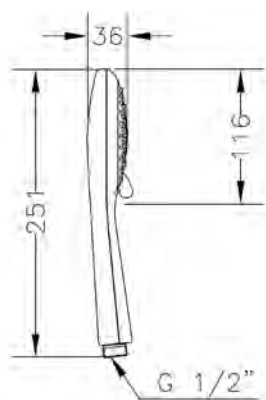
Ref.: DX03 45 Mango de ducha O3 jets (caja) O3 jets handshower (box)
