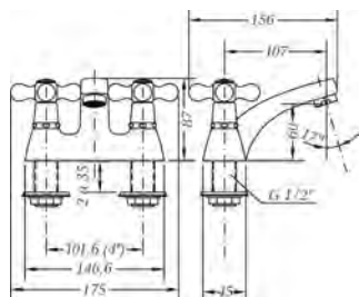
Ref.: 68511 09 45 66 Mezclador lavabo centerset 4" Wash-basin mixer 4" centerset
