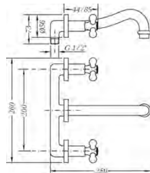
Ref.: 68131 09 45 66 Grupo de lavabo empotrado Built-in wash basin
