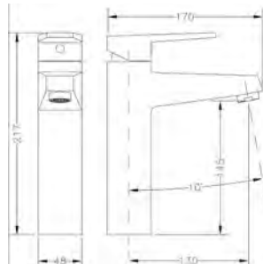
Ref.: 64134 04 45 66 Monomando de lavabo medio alto apertura en frío Medium high single lever wash-basin mixer cold start
