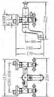
Ref.: 68526 09 43 66 Mezclador de baño bronce con kit Bath mixer bronze with kit
