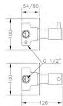
Ref.: 65114 30 45 66 Inversor cerámico 3 vías empotrado con placa cuadrada Built-in 3 way ceramic diverter With square plate
