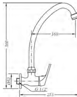
Ref.: 1005 04 Grifo mural con tubo alto 1 agua cartucho 25 1 water wall sink high spout 25 cartridge
