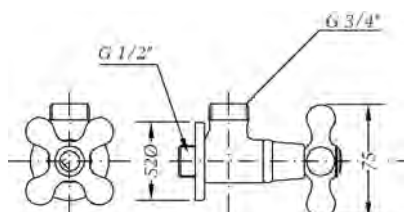
Ref.: 568575 45 Cuerpo grifo mural Wall tap
