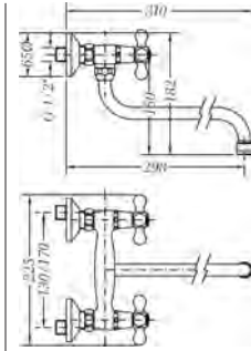
Ref.: 68550 09 45 66 Grupo mural fregadera 11 cm caño tubo alto 18cm Wall sink mixer 11cm high tube spout 18cm
