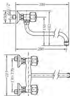
Ref.: 68197 11 45 66 Grupo mural fregadera 15cm caño tubo bajo 24cm Wall sink mixer 15cm low tube spout 24cm
