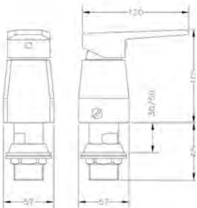
Ref.: 64142 16 45 66 Monomando de bidé con transmisión Single lever bidet mixer with diverter
