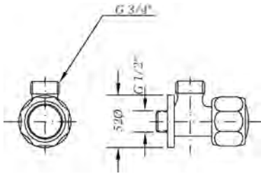
Ref.: 568083 45 Cuerpo grifo mural Wall tap
