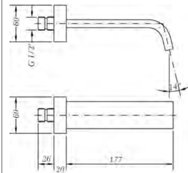
Ref.: 1674 45 Caño mural baño cuadrado Square wall bath spout
