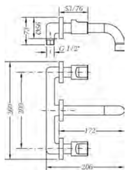
Ref.: 68131 07 45 66 Grupo de lavabo empotrado caño 16 cm Built-in wash basin with 16cm pipe
