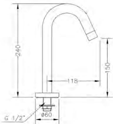
Ref.: 68917 45 Caño encimera inclinado tubo Sloping pipe spout
