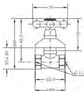
Ref.: 68590 09 45 66 Llave de paso 1/2" Stopcock 1/2"
