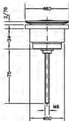
Ref.: 100205 45 Válvula click universal 1 1/4" 1 1/4" universal click valve
