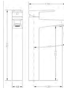
Ref.: 64136 04 45 66 Monomando de lavabo alto apertura en frío High single lever wash-basin mixer cold start
