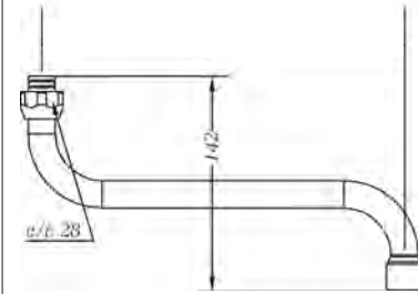
Ref.: 68904 45 Caño bajo tubo 24 cm Low tube spout 24 cm
