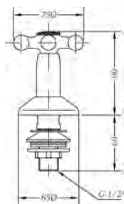
Ref.: 68520 09 45 66 Grifo bidé Bidet tap
