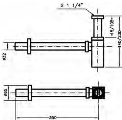
Ref.: 1621 07 Sifon botella para lavabo y bidé 1 1/4" 1 1/4" bidet and basin siphon
