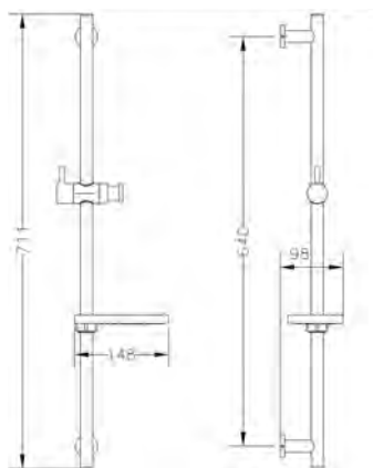
Ref.: 1639 45 Barra ducha metálica (caja) Metallic shower bar (box)
