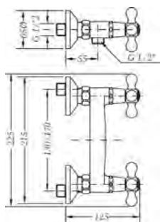
Ref.: 68530 09 45 66 Mezclador de ducha con kit Shower mixer with kit
