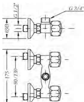
Ref.: 568195 45 Cuerpo grupo mural 11cm Wall mounted mixer 11cm
