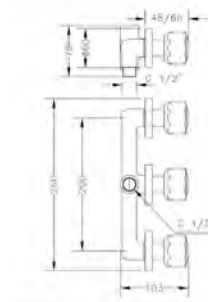
Ref.: 68116 11 45 66 Grupo baño empotrado 8" con inversor Built-in 8" bath mixer with diverter
