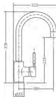
Ref.: 65203 18 45 66 Monomando de fregadera Single lever sink mixer
