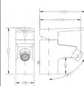
Ref.: 64140 14 45 66 Monomando de bidé Single lever bidet mixer
