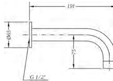
Ref.: 1668 45 Caño mural baño cilíndrico Round wall bath spout
