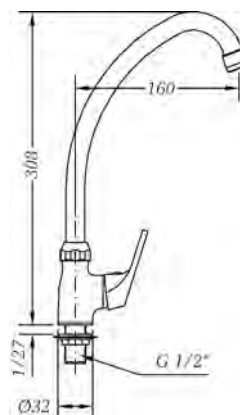
Ref.: 1009 04 Grifo fregadera 1 agua cartucho 25 1 water sink 25 cartridge
