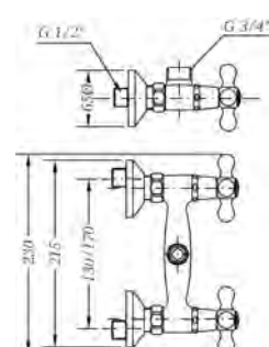
Ref.: 568555 45 Cuerpo grupo mural 15cm Wall mixer 15 cm
