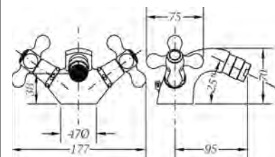
Ref.: 68515 09 45 66 Monobloc de bidé Bidet mixer
