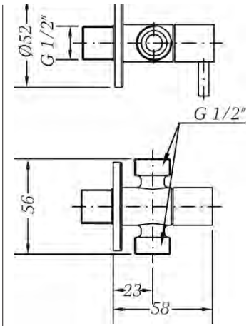
Ref.: 3108 04 Válvula de escuadra doble 1/2" - 1/2" ducha-inodoro Inox Inox double angle valve 1/2" - 1/2" shower-WC
