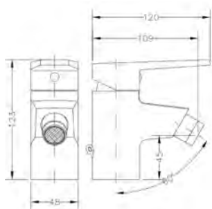
Ref.: 64140 04 45 66 Monomando de bidé apertura en frío Single lever bidet mixer cold start
