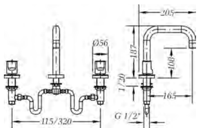
Ref.: 68120 07 45 66 Batería de lavabo caño recto Widespread wash basin mixer with straight pipe
