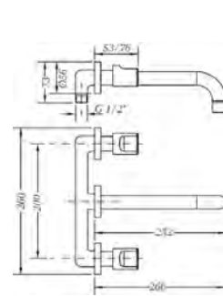
Ref.: 68132 08 45 66 Grupo de lavabo empotrado caño 22cm Built-in wash basin with 22cm pipe
