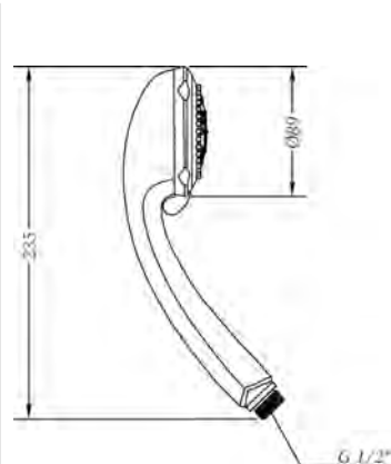
Ref.: DXE5 45 Mango de ducha E5 jets (caja) E5 jets handshower (box)
