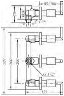
Ref.: 68116 12 45 66 Grupo baño empotrada 8" con inversor Built-in 8" bath mixer with diverter
