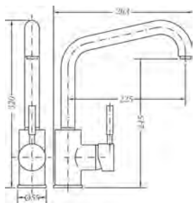
Ref.: 65204 18 45 66 Monomando de fregadera Single lever sink mixer
