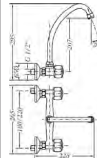
Ref.: 68103 11 45 66 Grupo mural fregadera 20 cm caño tubo alto vertical Wall sink mixer 20cm swan neck spout
