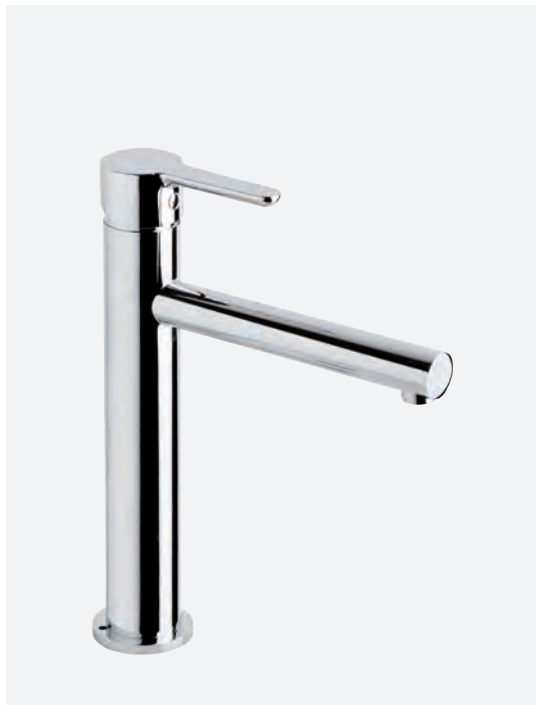
Ref.: 65134 19 45 66 Monomando de lavabo medio alto Medium high single lever wash-basin mixer. Cartucho 2 posiciones | 2-position cartridge
