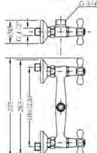
Ref.: 568565 45 Cuerpo grupo mural 20cm Wall mixer 20 cm
