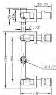
Ref.: 68115 07 45 66 Grupo ducha empotrada 8\"/> Built-in shower 8\" shower mixer
