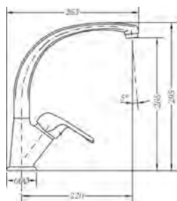
Ref.: 61210 06 45 66 Monomando de fregadera caño fundido Single lever sink mixer casted spout
