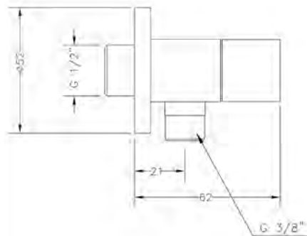
Ref.: 3106 04 Válvula de escuadra cuadrada 3/8\"/>
