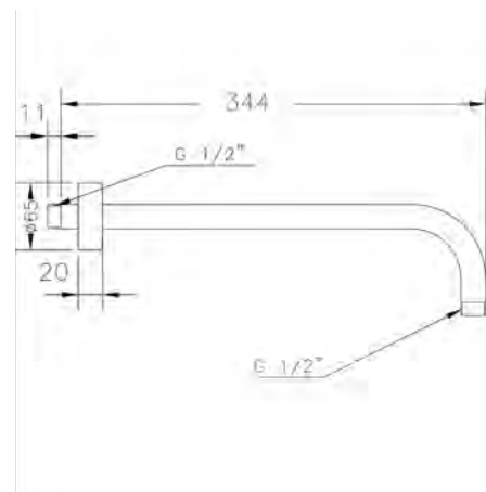
Ref.: B65113 18 Brazo pared redondo 35 cm Round arm 35 cm
