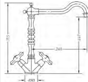
Ref.: 68595 09 45 66 Monobloc de fregadera cromo Sink mixer chromed
