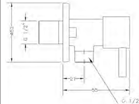
Ref.: 3104 05 Válvula de escuadra redonda 1/2\"/>
