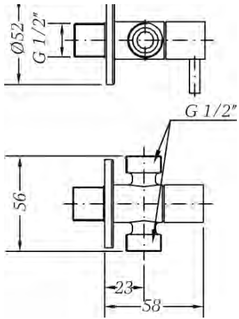
Ref.: 3107 04 Válvula de escuadra doble 1/2" - 1/2" ducha-inodoro Double angle valve 1/2" - 1/2" shower-WC
