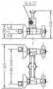
Ref.: 68531 09 45 66 Mezclador de ducha cromo con kit Shower mixer chromed with kit
