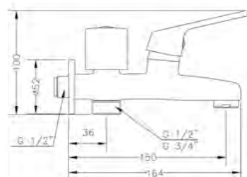
Ref.: 1024 04 Grifo doble combinable a 1/2\"- 3/4\" y atomizador Double outlet tap 1/2\" - 3/4\" and aerator
