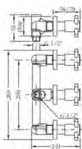
Ref.: 68116 08 45 66 Grupo baño empotrada 8" con inversor Built-in 8" bath mixer with diverter
