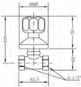
Ref.: 68170 11 45 66 Llave de paso 1/2" Stopcock 1/2"
