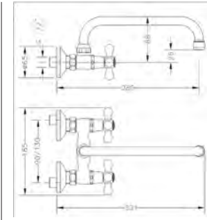
Ref.: 68196 09 45 66 Grupo mural fregadera 11 cm caño tubo alto 24cm Wall sink mixer 11cm high tube spout 24cm
