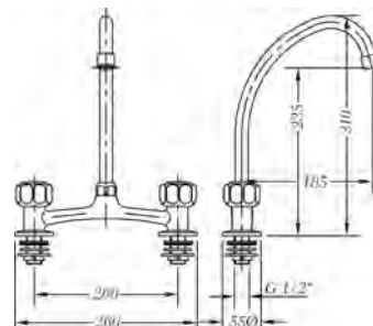
Ref.: 68199 11 45 66 Mezclador mesada 8" caño tubo Mixer mesada 8" swan neck spout
