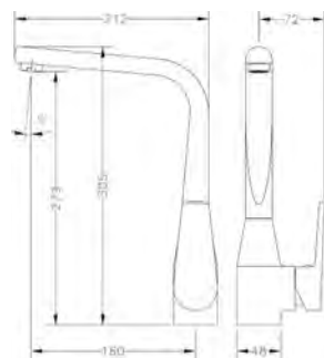
Ref.: 64201 04 45 66 Monomando de fregadera apertura en frío Single lever sink mixer cold start
