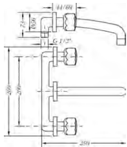
Ref.: 68131 11 45 66 Grupo de lavabo empotrado Built-in wash basin
