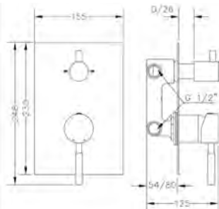
Ref.: 65117 18 45 66 Monomando empotrado con inversor cerámico 2 vías Built-in single handle mixer with 2 way ceramic diverter
