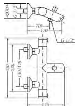
Ref.: 67102 14 45 67 Termostática baño Thermostatic bath
