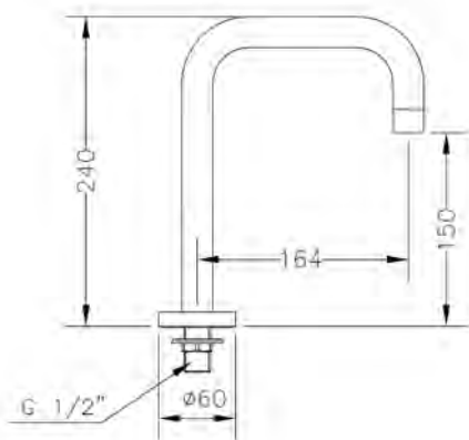
Ref.: 68915 45 Caño encimera recto tubo Straight pipe spout
