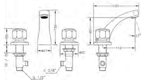
Ref.: 68120 11 45 66 Batería de lavabo Widespread wash basin mixer
