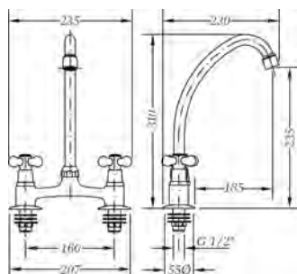
Ref.: 68194 09 45 66 Mezclador mesada 6" caño tubo Mixer mesada 6" swan neck spout
