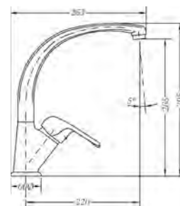
Ref.: 61204 06 45 66 Monomando de fregadera caño conformado Single-lever sink mixer tube spout
