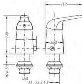
Ref.: 61142 06 45 66 Monomando de bidé con transmisión Single lever bidet mixer with diverter
