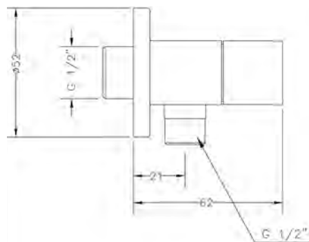
Ref.: 3106 05 Válvula de escuadra cuadrada 1/2\"/>
