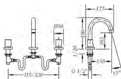
Ref.: 68124 07 45 66 Batería de lavabo caño cisne Widespread wash basin mixer with swan neck pipe
