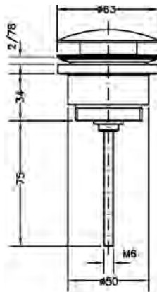
Ref.: 100211 45 Válvula click "Luxe" 1 1/4" 1 1/4" "Luxe" click valve
