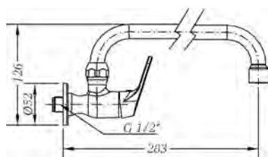
Ref.: 1008 04 Grifo mural con tubo 24 cm 1 agua cartucho 25 1 water wall sink spout 24cm 25 cartridge
