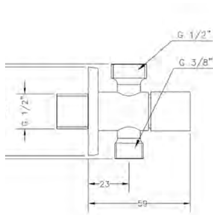
Ref.: 3108 03 Válvula de escuadra doble 1/2" - 3/8" ducha-inodoro Inox Inox double angle valve 1/2" - 3/8" shower-WC
