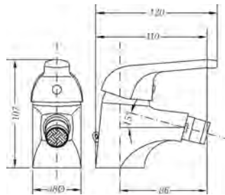
Ref.: 60140 06 45 66 Monomando de bidé Single lever bidet mixer
