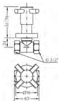
Ref.: 68170 08 45 66 Llave de paso 1/2" Stopcock 1/2"
