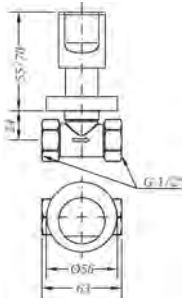
Ref.: 68170 07 45 66 Llave de paso 1/2" Stopcock 1/2"
