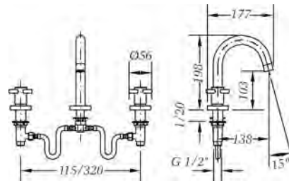
Ref.: 68124 08 45 66 Batería de lavabo caño cisne Widespread wash basin mixer with swan neck pipe
