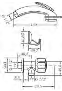
Ref.: 68001 11 45 66 Grifo de bide con teleducha Bidet tap with shower
