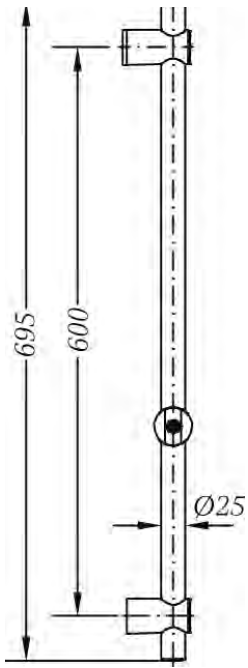
Ref.: 1748 45 Conjunto Tau, barra, flexo y ducha 5 jets (caja) Tau set, bar, hose and 5 jets handshower (box)
