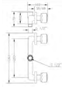
Ref.: 68115 11 45 66 Grupo ducha empotrado 8" Built-in 8" shower mixer
