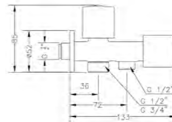
Ref.: 1023 04 Grifo doble combinable 1/2\"-3/4\" y 1/2\" Double outlet tap 1/2\" - 3/4\" and 1/2\"
