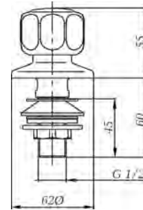
Ref.: 68160 11 45 66 Grifo bidé Bidet tap
