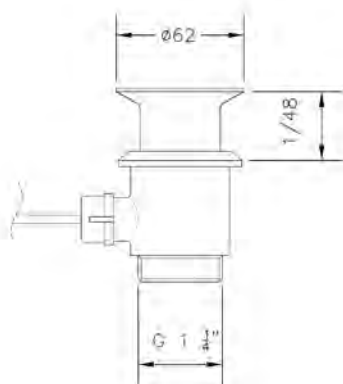
Ref.: 100200 45 Válvula automática plástico 1 1/4" 1 1/4" Plastic automatic valve
