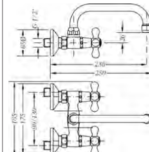
Ref.: 68560 09 45 66 Grupo mural fregadera 15cm caño tubo bajo 24cm Wall sink mixer 15cm low tube spout 24cm
