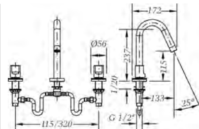
Ref.: 68125 07 45 66 Batería de lavabo caño inclinado Widespread wash basin mixer with sloping pipe
