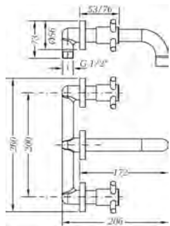
Ref.: 68131 08 45 66 Grupo de lavabo empotrado caño 16cm Built-in wash basin with 16cm pipe
