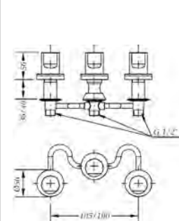
Ref.: 68142 07 45 66 Batería de bidé con transmisión Widespread bidet mixer with transmission
