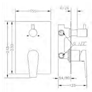
Ref.: 64118 04 45 66 Monomando empotrado con inversor cerámico 3 vías Built-in single handle mixer with 3 way ceramic diverter
