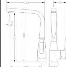
Ref.: 64201 14 45 66 Monomando de fregadera Single lever sink mixer
