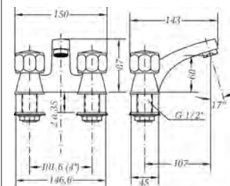
Ref.: 68122 11 45 66 Mezclador lavabo centerset 4" Wash-basin mixer 4" centerset
