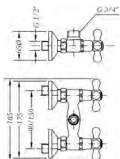
Ref.: 568550 45 Cuerpo grupo mural 11 cm Wall mixer 11 cm
