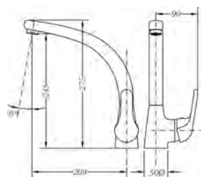
Ref.: 61203 06 45 66 Monomando de fregadera caño conformado Single-lever sink mixer tube spout
