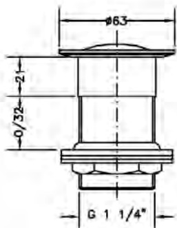
Ref.: 100207 45 Válvula click 1 1/4" 1 1/4" click valve
