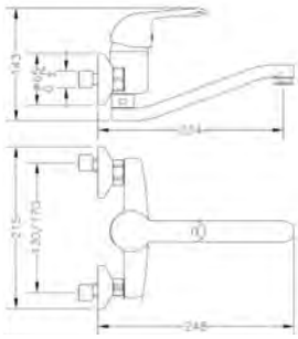
Ref.: 61196 06 45 66 Monomando de fregadera caño inferior elevado Wall single lever sink mixer low spout
