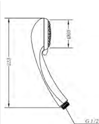
Ref.: DXE2 45 Mango de ducha E2 jets (caja) E2 jets handshower (box)
