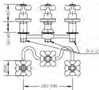
Ref.: 68142 09 45 66 Batería de bidé con transmisión Widespread bidet mixed with transmission
