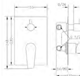
Ref.: 64117 04 45 66 Monomando empotrado con inversor cerámico 2 vías Built-in single handle mixer with 2 way ceramic diverter
