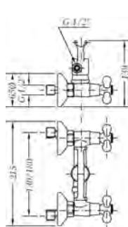
Ref.: 68531 09 43 66 Mezclador de ducha bronce con kit Shower mixer bronze with kit
