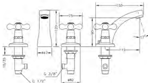
Ref.: 68510 09 45 66 Batería lavabo Widespread wash basin mixer
