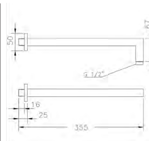
Ref.: B63113 26 Brazo pared cuadrado 35 cm Square wall arm 35 cm
