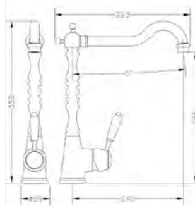
Ref.: 68201 39 45 66 Monomando de fregadera cromo cartucho 40 Sink mixer chromed 40 cartridge
