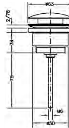
Ref.: 100211 43 Válvula click "Luxe" bronce 1 1/4" 1 1/4" "Luxe" click valve bronze
