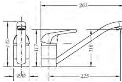
Ref.: 61200 06 45 66 Monomando de fregadera Single lever sink mixer
