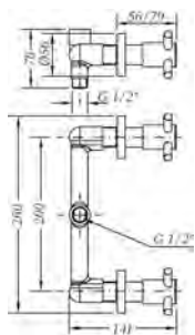
Ref.: 68115 08 45 66 Grupo ducha empotrada 8" Built-in 8" shower mixer
