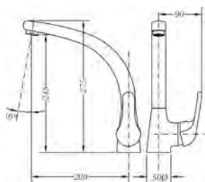
Ref.: 61201 06 45 66 Monomando de fregadera caño fundido Single lever sink mixer casted spout
