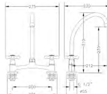
Ref.: 68545 09 45 66 Mezclador mesada 8" caño tubo Mixer mesada 8" swan neck spout
