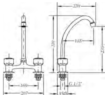
Ref.: 68194 11 45 66 Mezclador mesada 6" caño tubo Mixer mesada 6" swan neck spout
