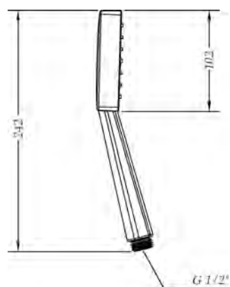
Ref.: DXK1 45 Mango de ducha K1 jets (caja) K1 jet handshower (box)
