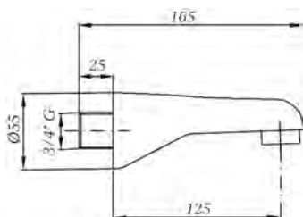
Ref.: 1667 45 Caño mural baño fundido Casted wall bath spout
