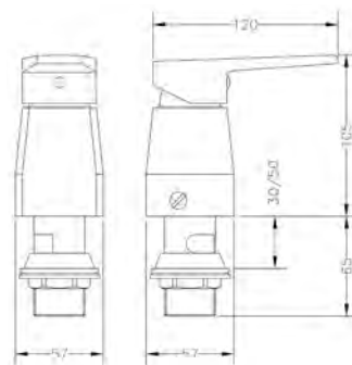
Ref.: 64142 04 45 66 Monomando de bidé con transmisión Single lever bidet mixer with diverter
