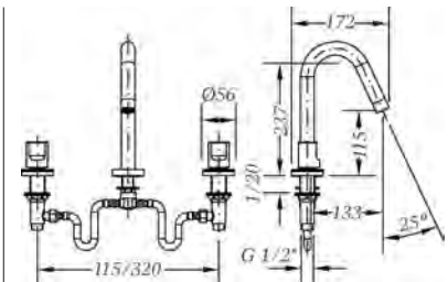
Ref.: 68125 08 45 66 Batería de lavabo caño inclinado Widespread wash basin mixer with sloping pipe
