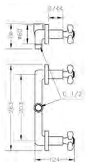
Ref.: 68535 09 45 66 Grupo ducha empotrado 8" Built-in 8" shower mixer
