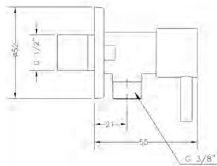
Ref.: 3104 04 Válvula de escuadra redonda 3/8\"/>
