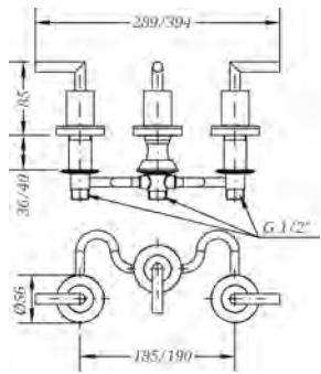
Ref.: 68142 12 45 66 Batería de bidé con transmisión Widespread bidet mixer with transmission
