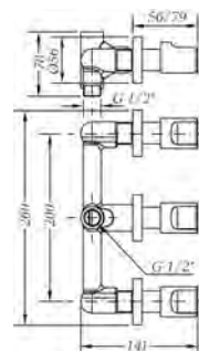
Ref.: 68116 07 45 66 Grupo baño empotrado 8\"/> Built-in 8\" bath mixer with diverter
