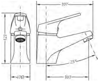
Ref.: 61130 22 45 66 Monomando de lavabo Plus Single lever Plus wash-basin mixer
