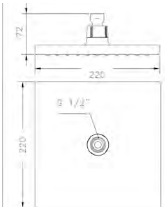
Ref.: R63112 26 Rociador cuadrado 22 cm Square shower head 22 cm
