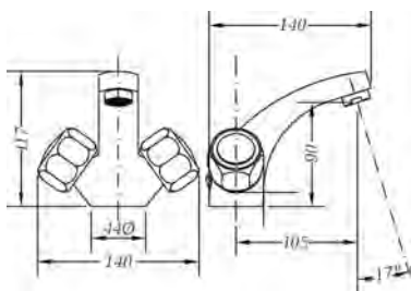
Ref.: 68130 11 45 66 Monobloc de lavabo Wash basin mixer
