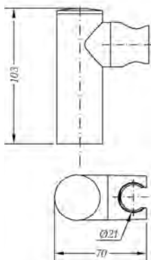
Ref.: 100153 45 Soporte ducha cilíndrico Cylindrical shower holder
