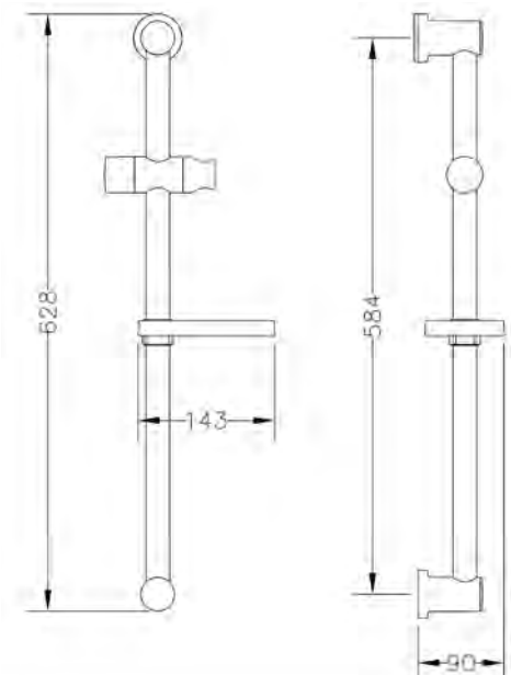
Ref.: 1638 45 Barra ducha redonda (caja) Round shower bar (box)
