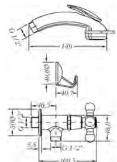
Ref.: 68001 09 45 66 Grifo de bide con teleducha Bidet tap with shower
