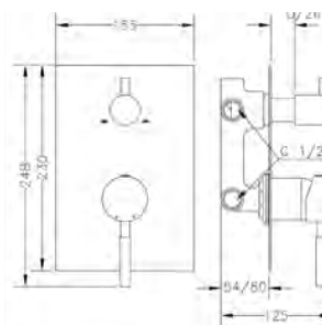
Ref.: 65118 18 45 66 Monomando empotrado con inversor cerámico 3 vías Built-in single handle mixer with 3 way ceramic diverter
