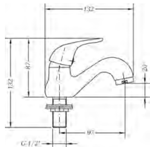
Ref.: 1007 04 Grifo lavabo 1 agua cartucho 25 1 water wash basin cartridge 25
