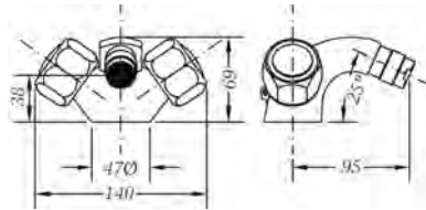
Ref.: 68140 11 45 66 Monobloc de bidé Bidet mixer
