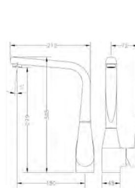
Ref.: 64201 16 45 66 Monomando de fregadera Single lever sink mixer
