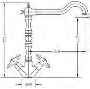
Ref.: 68595 09 43 66 Monobloc de fregadera bronce Sink mixer bronze
