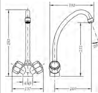
Ref.: 68200 11 45 66 Monobloc de fregadera caño tubo Sink mixer swan neck spout
