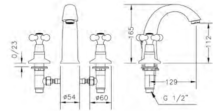
Ref.: 68120 09 45 66 Batería lavabo Widespread wash basin mixer
