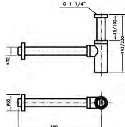
Ref.: 1622 07 Sifon botella para lavabo y bidé 1 1/4" 1 1/4" bidet and basin siphon
