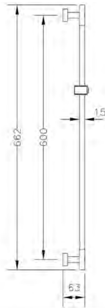
Ref.: 1637 45 Barra ducha Kenjo (caja) Kenjo shower bar (box)
