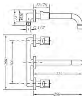
Ref.: 68132 07 45 66 Grupo de lavabo empotrado caño 22 cm Built-in wash basin with 22cm pipe
