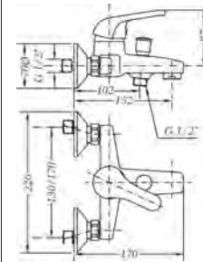
Ref.: 60100 06 45 66 Monomando de baño con kit Single lever bath mixer with kit
